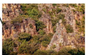
▲ Gneiss du Tanneron.
